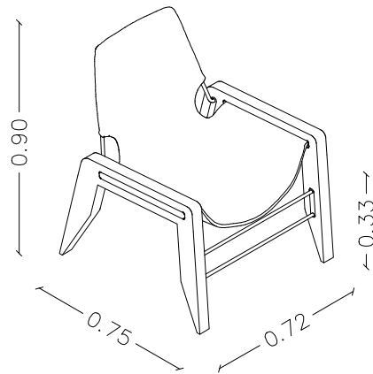
ISOMÉTRICA
