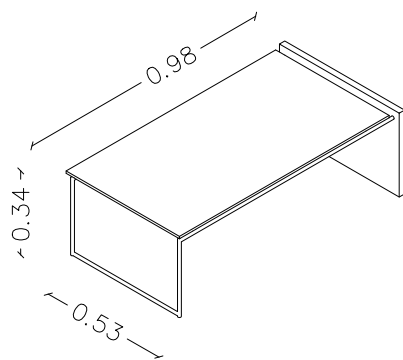
ISOMÉTRICA
